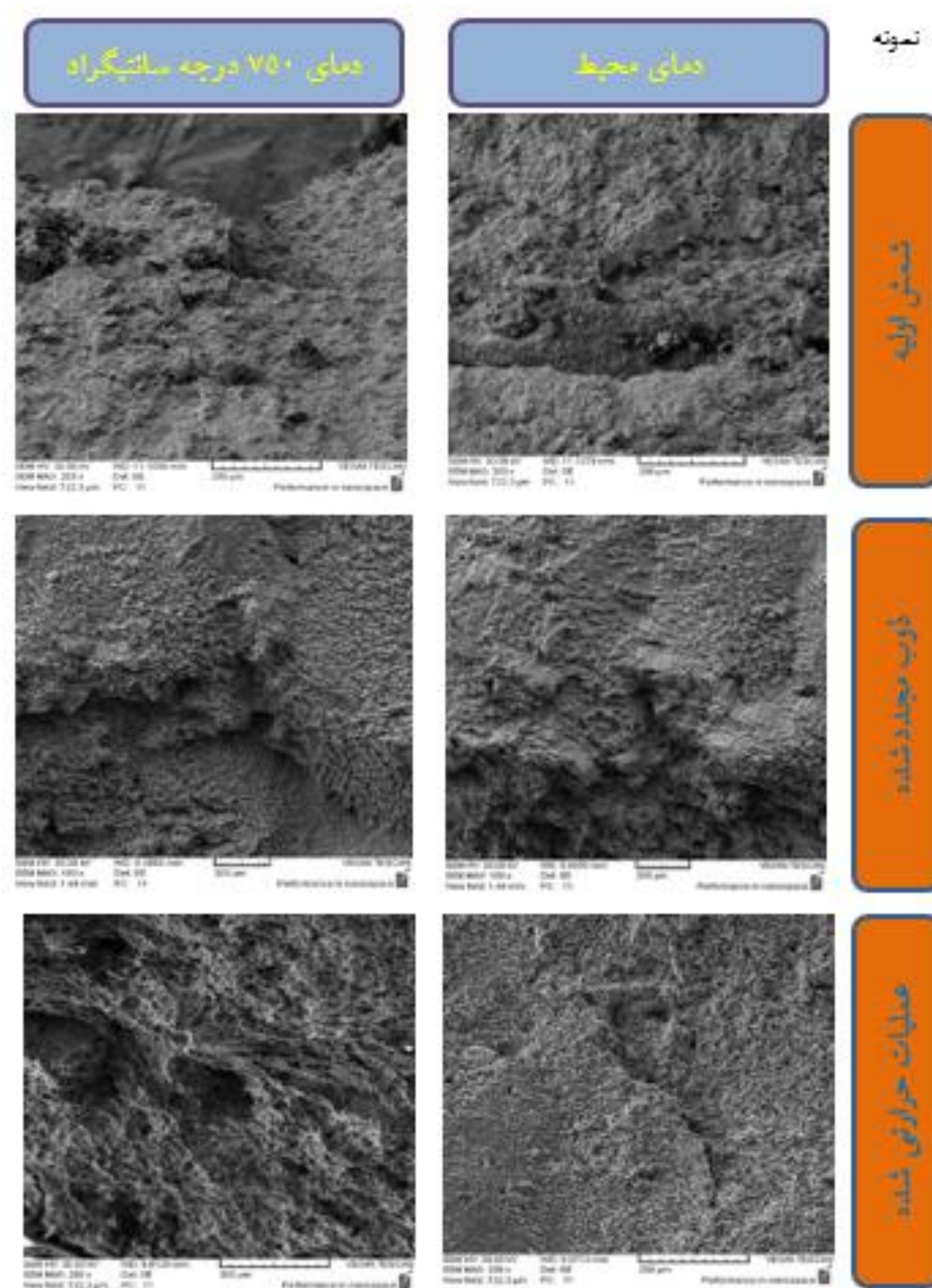
شکل ۸- تصاویر FESEM سطوح شکست نمونه‌ها در دو دمای محیط و ۷۵۰ درجه سانتی‌گراد.
