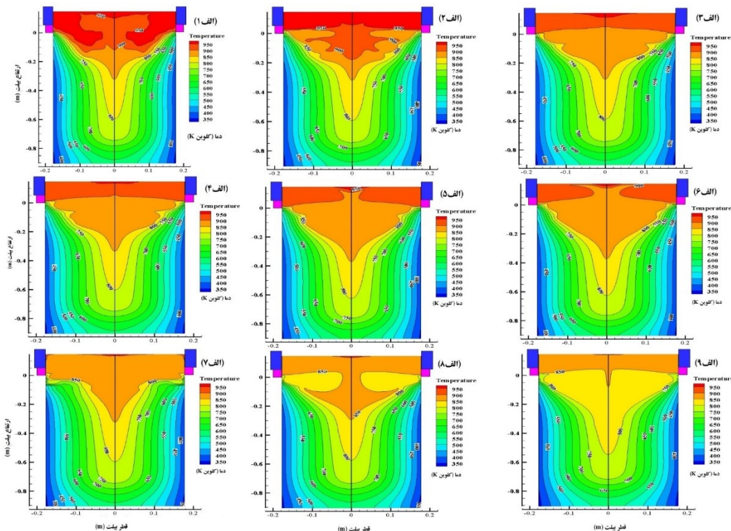
شکل ۲- پروفیل‌های دما (کلوین) برحسب آمپر-دور بالاپوش: (الف) DC، (ب) ۹۶۰۰ آمپر-دور، (ج) ۱۲۰۰۰ آمپر-دور، (د) ۱۴۴۰۰ آمپر-دور، (ه) ۱۹۲۰۰ آمپر-دور، (و) ۲۴۰۰۰ آمپر-دور، (ز) ۳۰۰۰۰ آمپر-دور، (ح) ۳۶۰۰۰ آمپر-دور و (ط) ۴۸۰۰۰ آمپر-دور.
