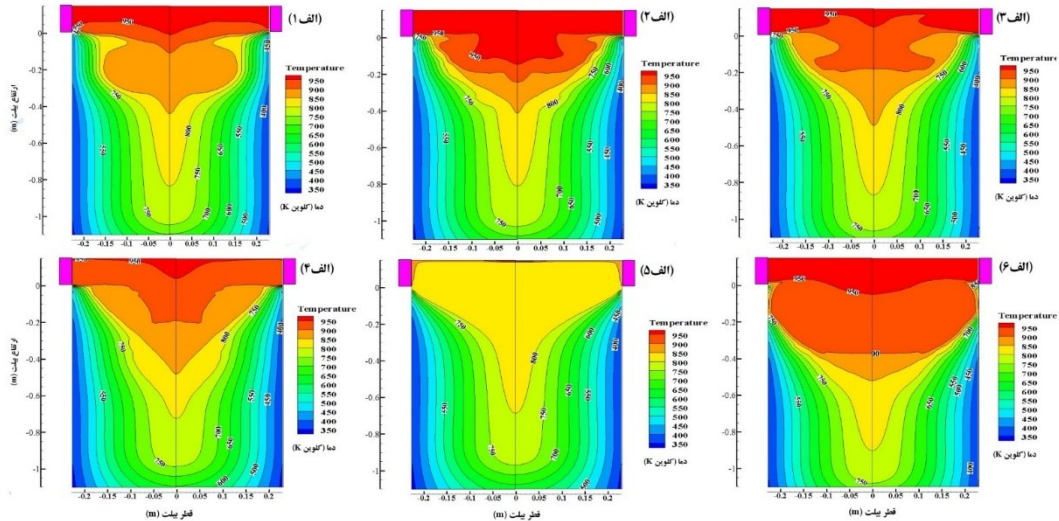
شکل ۳- پروفیل‌های دما (کلون) برحسب آمپر-دور در قالب بدون بالابوش: (الف) DC، (ب) ۹۶۰۰ آمپر-دور، (ج) ۱۲۰۰۰ آمپر-دور، (د) ۱۴۴۰۰ آمپر-دور، (ه) ۱۹۲۰۰ آمپر-دور و (ف) ۲۴۰۰۰ آمپر-دور.
