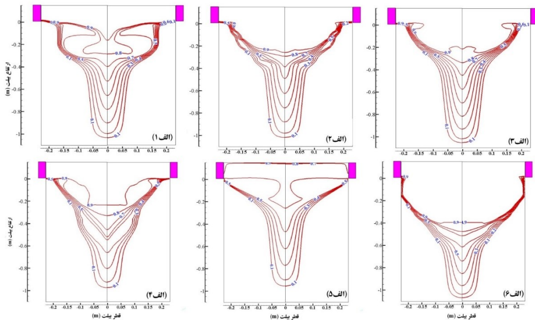
شکل ۹- پروفیل‌های کسر جامدبر حسب آمپر- دور در قالب بدون بالاپوش: (الف) DC، (ب) ۹۶۰۰ آمپر-دور، (ج) ۱۲۰۰۰ آمپر-دور، (د) ۱۴۴۰۰ آمپر-دور، (ه) ۱۹۲۰۰ آمپر-دور و (و) ۲۴۰۰۰ آمپر-دور.
