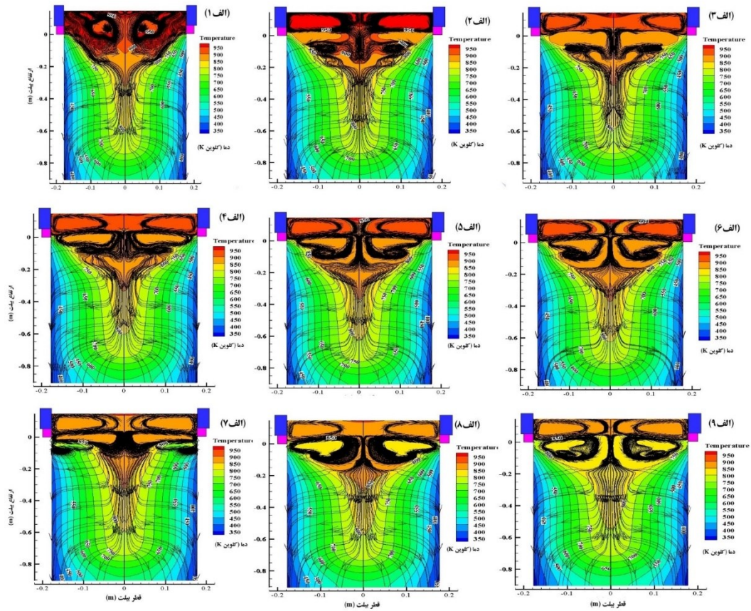
شکل ۴- پروفیل‌های جریان برحسب آمپر-دور در قالب بالابوش: (الف) DC، (ب) ۹۶۰۰ آمپر-دور، (ج) ۱۲۰۰۰ آمپر-دور، (د) ۱۴۴۰۰ آمپر-دور، (ه) ۱۹۲۰۰ آمپر-دور، (و) ۲۴۰۰۰ آمپر-دور، (ز) ۳۰۰۰۰ آمپر-دور، (ح) ۳۶۰۰۰ آمپر-دور و (ی) ۴۸۰۰۰ آمپر-دور.
