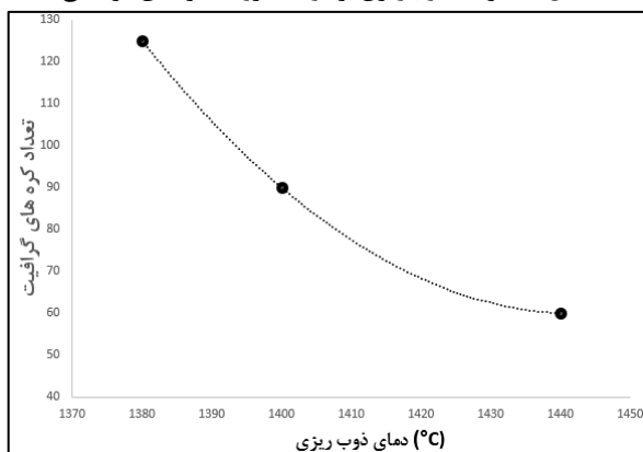
شکل ۱۰- اثر دما ذوب‌ریزی بر تعداد کره‌های گرافیتی
