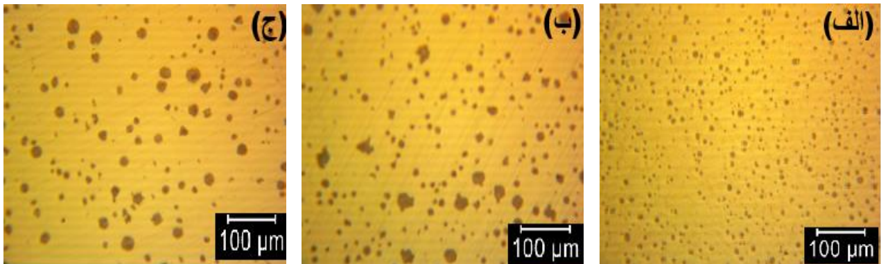
شکل ۸- تصاویر متالوگرافی از شمش‌های ریخته‌گری شده در دماهای مختلف الف) ۱۳۸۰ (ب) ۱۴۰۰ و ج) ۱۴۴۰°C
