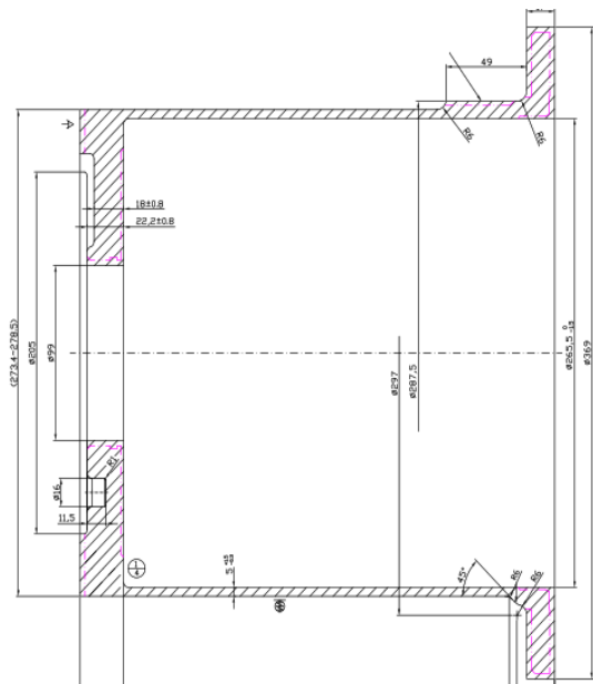
شکل ۱. نقشه مهندسی قطعه پوسته زنگوله (واحد: میلی‌متر)
