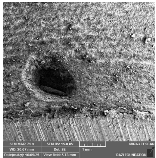
شکل ۵- تصویر SEM از عیب کشیدگی میکرو
