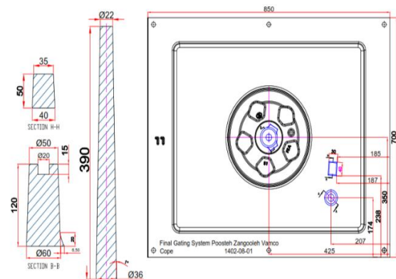
شکل ۲- سیستم راهگاهی مورد استفاده در ریخته‌گری قطعه زنگوله
