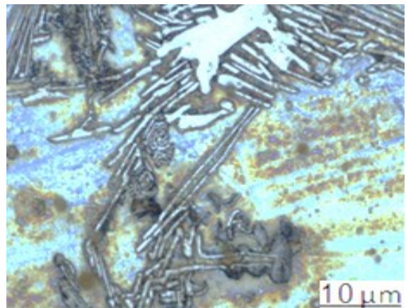
شکل ۵- تصویر میکروسکوپی نوری از ریزساختار ریختگی. نمونه A (محلول اچ نیپال ۳ درصد)
