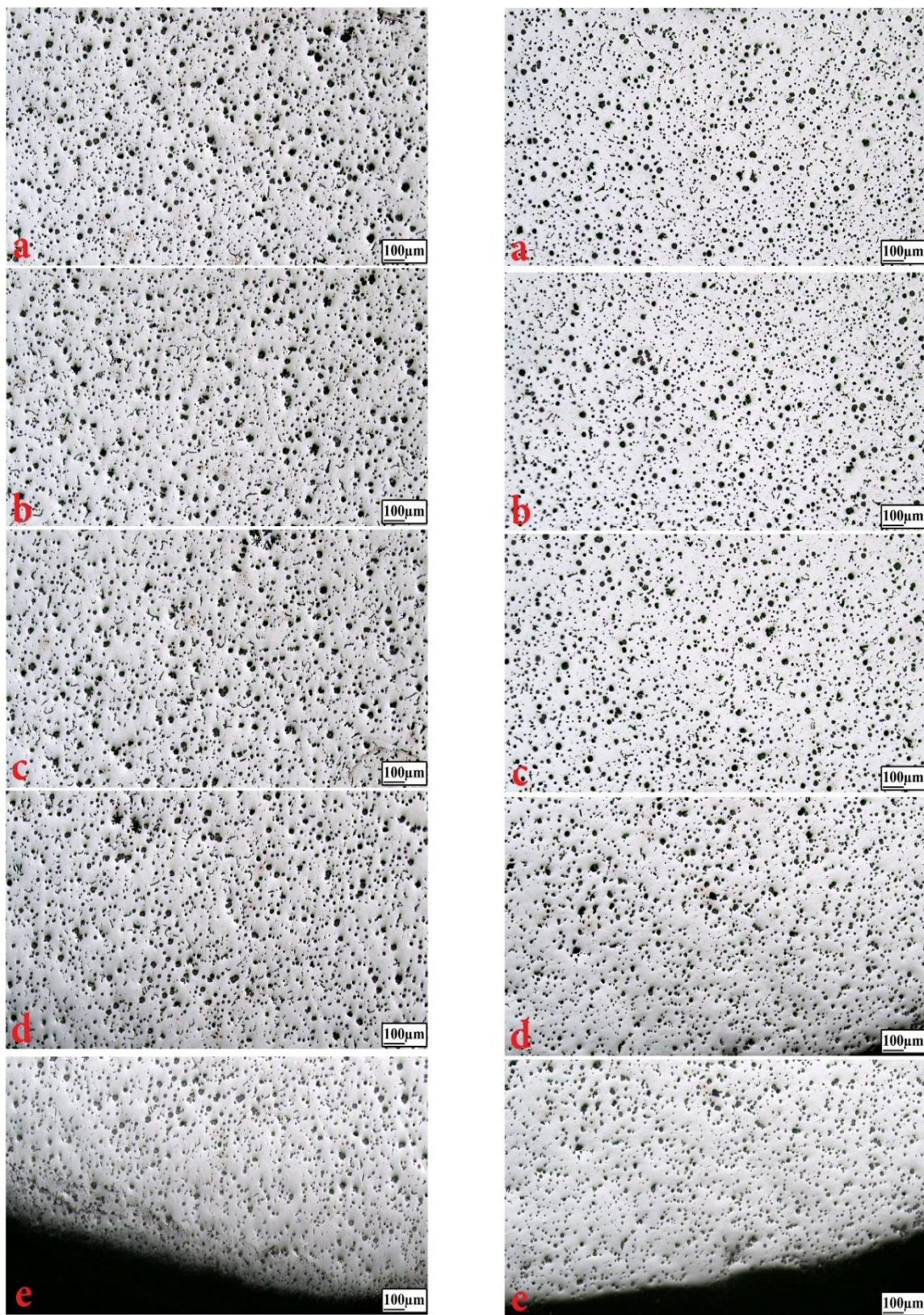
شکل ۸- ریز ساختار مرکز تا لبه میله ریخته شده در دمای ۱۴۴۰ °C: الف) مقطع شماره ۱ (قسمت بالا و دورترین فاصله از راهباره)، ب) مقطع شماره ۲ (مقطع میانی). تصاویر از a تا e به ترتیب مرکز تا لبه مقطع را نشان می‌دهد.
