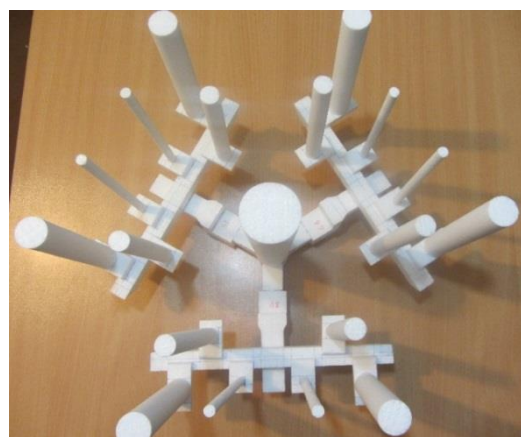
شکل ۲- تصویر مدل فومی ساخته شده و اجزای مربوط به آن.
