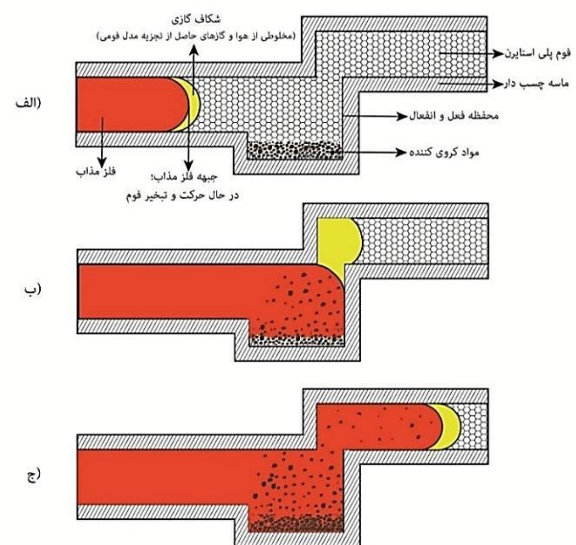
شکل ۵- مراحل پر کردن قالب در روش منیزیم در راهگاه- توپر: (الف) ورود مذاب از راهگاه به راهبار در حال تبخیر فوم پلی استایرین، (ب) مذاب در حال واکنش با مواد کروی کننده، (ج) مذاب واکنش کرده با مواد کروی کننده و در حال پر کردن قسمت های قالب پس از خروج از محفظه و واکنش.
