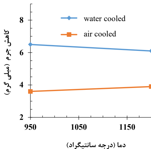
شکل ۱۱- ارتباط بین دمای بارریزی و کاهش جرم بر اثر سایش
