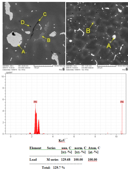
شکل ۹- تصاویر SEM و طیف تفکیک انرژی فاز سرب خالص (فاز A)
