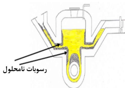
شکل ۱- تصویر نمادین از کوره‌ی ذوب‌ریز فشاری [۷].
