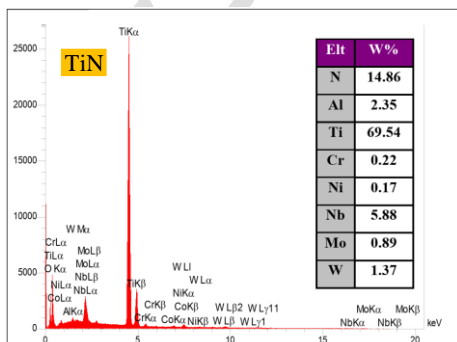
شکل ۴- تصویر میکروسکوپ الکترونی روبشی و نتایج آنالیز EDS از ذرات فاز ثانویه پس از همگن‌سازی در دمای ۱۱۰۰ درجه سانتیگراد به مدت ۱۰ ساعت و ب) همگن‌سازی در دمای ۱۱۶۰ درجه سانتیگراد به مدت ۱۰ ساعت.
