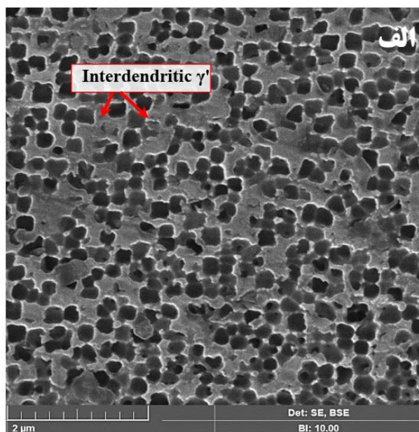
شکل ۲- تصاویر میکروسکوپ الکترونی روبشی از رسوبات \gamma' در ریزساختار نمونه ریخته‌گری M647 پس از ذوب مجدد در کوره VAR (الف) مناطق بین دندریتی (ب) هسته دندریتی.
