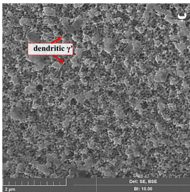
شکل ۲- تصاویر میکروسکوپ الکترونی روبشی از رسوبات \gamma' در ریزساختار نمونه ریخته‌گری M647 پس از ذوب مجدد در کوره VAR (الف) مناطق بین دندریتی (ب) هسته دندریتی.
