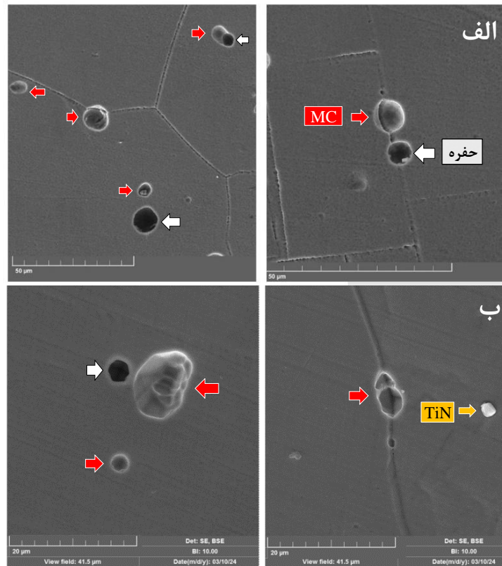
شکل ۴- تصویر میکروسکوپ الکترونی روبشی و نتایج آنالیز EDS از ذرات فاز ثانویه پس از همگن‌سازی در دمای ۱۱۰۰ درجه سانتیگراد به مدت ۱۰ ساعت و ب) همگن‌سازی در دمای ۱۱۶۰ درجه سانتیگراد به مدت ۱۰ ساعت.
