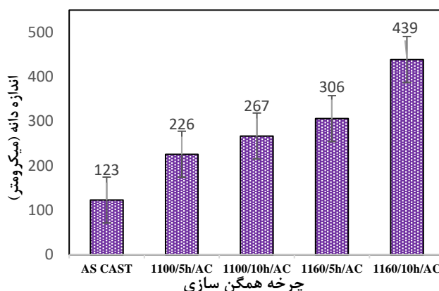
شکل ۵ - تاثیر چرخه همگن‌سازی بر اندازه دانه سوپرآلیاژ M647.
